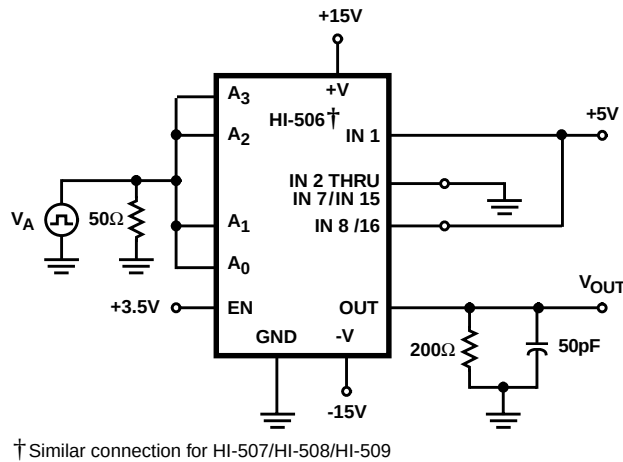
FIGURE 9A. TEST CIRCUIT
