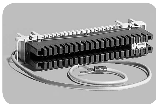
LSA PROFIL®-Erddrahtleiste 2/34
