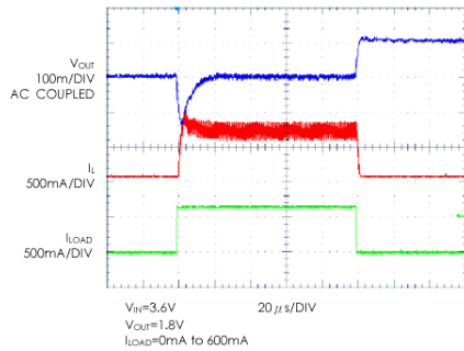
Fig. 16: Load Step
