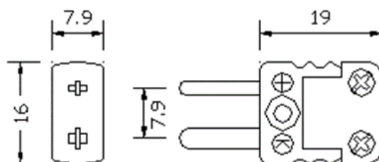
Miniature Plug
