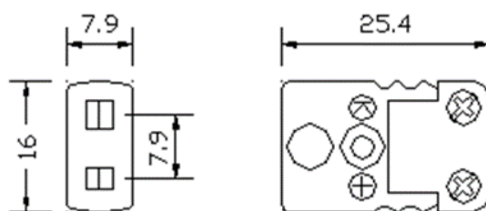
Miniature Socket
