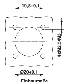
Einbaumaße
