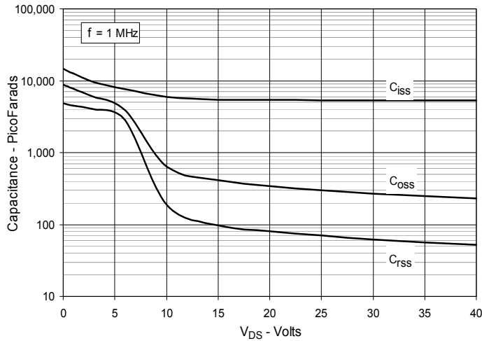
Fig. 13. Capacitance
