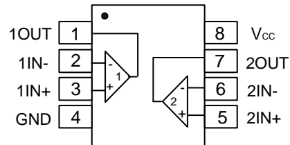
SO-8/TSSOP-8/MSOP-8
