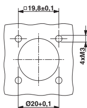
Einbaumaße: RF-1.S..8AA.00, RF-1.P..8AA.00
