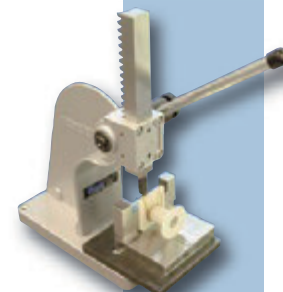
Manual Arbor Press
