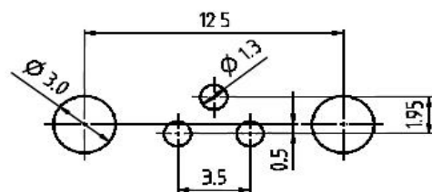
Leiterplattenbohrbild
