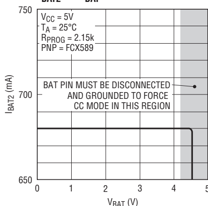
IBAT2 vs VBAT
