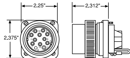
Style SKWM
