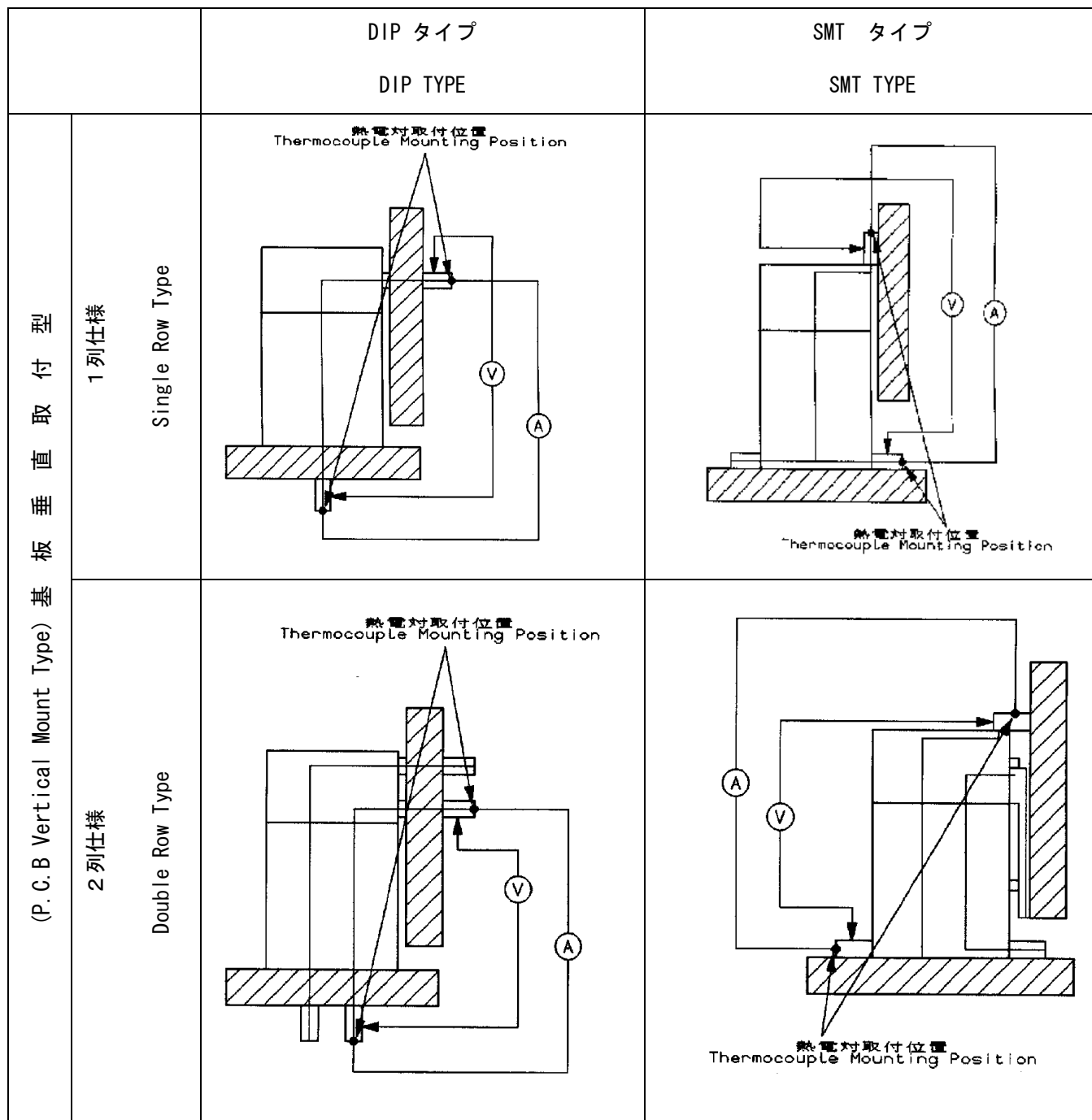
Fig. 6 (1/2) ローレベル総合抵抗測定方法
