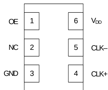
Si531 LVDS/LVPECL/CML
