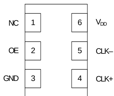
Si530 LVDS/LVPECL/CML
