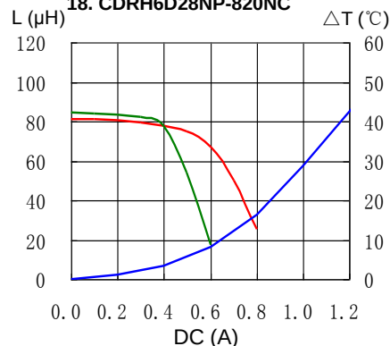
18. CDRH6D28NP-820NC
