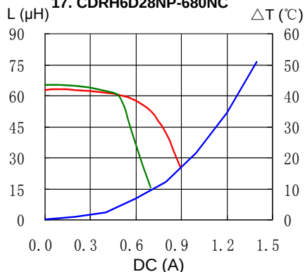
17. CDRH6D28NP-680NC
