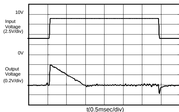
S-8520C30MC (Iout:10mA)
