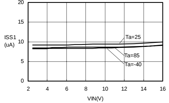
ISS1-VIN S-8520/21(Fosc:60kHz)
