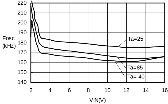
Fosc-VIN S-8520/21(Fosc:180kHz)
