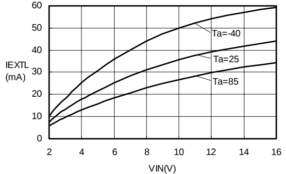
IEXTL-VIN S-8520/21
