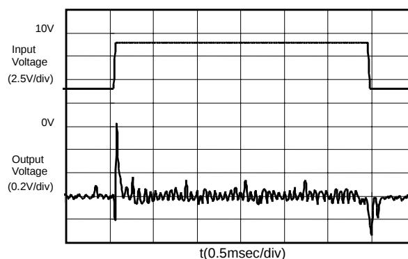
S-8520C30MC (Iout:500mA)
