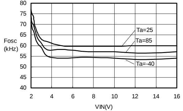
Fosc-VIN S-8520/21(Fosc:60kHz)
