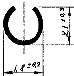
DRAHTPRESSHÜLSE
