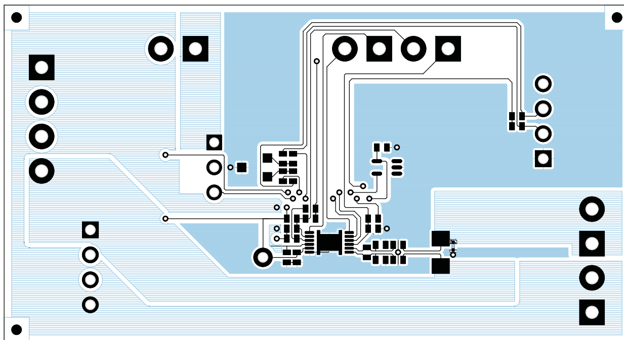
Figure 20. Top Layer
