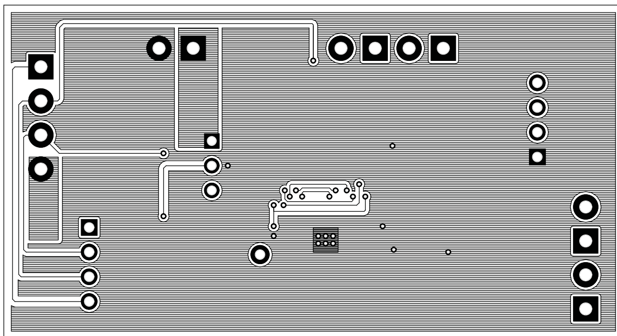
Figure 21. Bottom Layer
