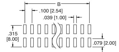
PH2-26-UA-SMT
