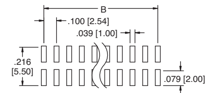
PH2-20-UA-SMT
