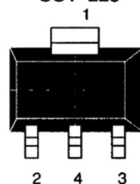
SOT-223
