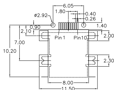
P.C.Board Layout Type 5
