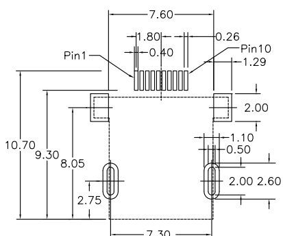
P.C.Board Layout Type 4
