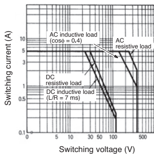
G2R-1Z, G2R-1AZ
