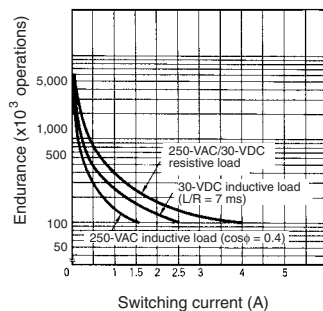
G2R-24, G2R-2A4
