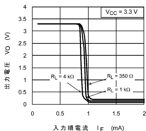
図 12.2.6 V_O - I_F
