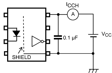
図 12.1.3 I_{CCH} 測定回路
