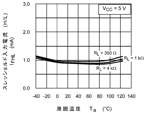
図 12.2.7 I_{FHL} - T_a
