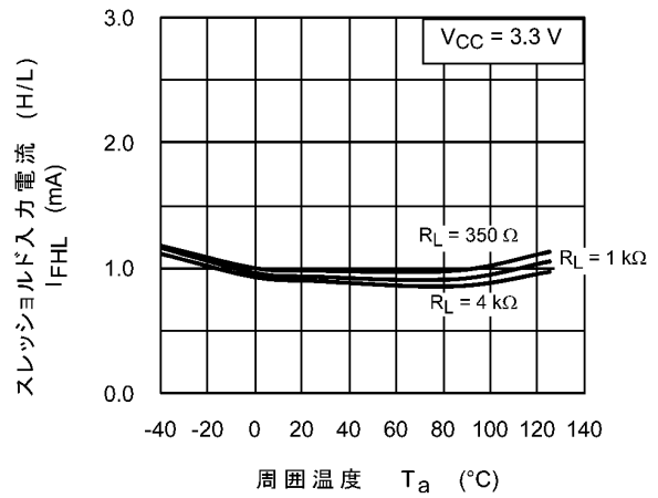
図 12.2.8 I_{FHL} - T_a
