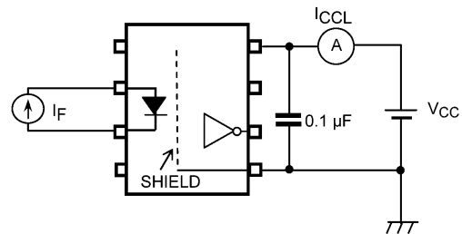
図 12.1.4 I_{CCL} 測定回路
