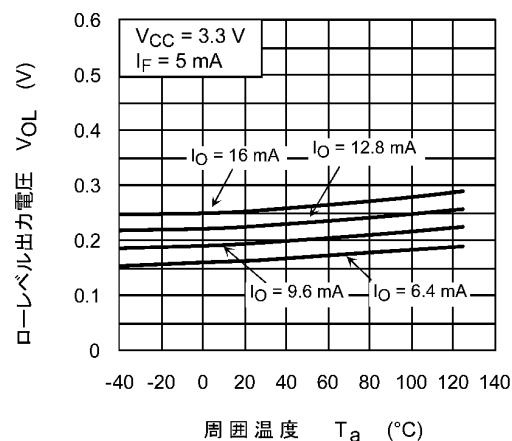
図 12.2.4 V_{OL} - T_a
