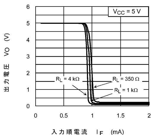
図 12.2.5 V_O - I_F
