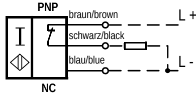
3RG40130AF01:
