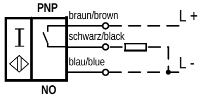
3RG40130AG01:
