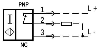
3RG40133AF01:
