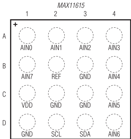
WLP
