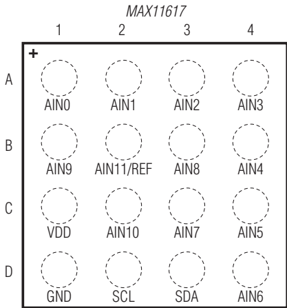
WLP
