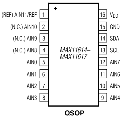
QSOP
