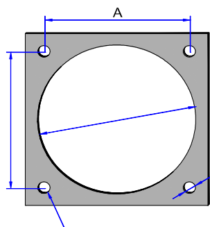
Lochbild 1 Steckmontage
