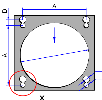
Lochbild 4 Steck-Schubmontage
