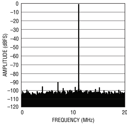
LTC2257-14: 8k Point FFT, f_{IN} = 69\text{MHz} , -1\text{dBFS} , 40\text{MSPs}
