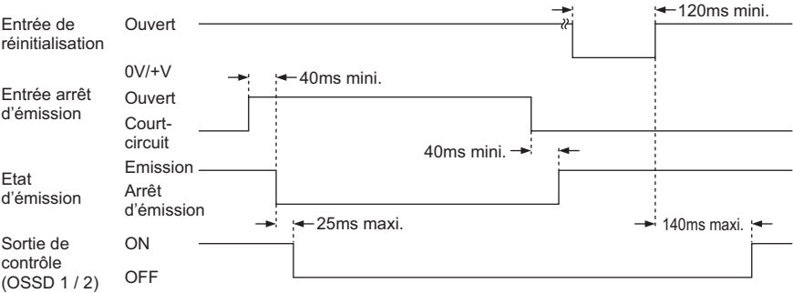
Chronogramme dans le cas d’une réinitialisation manuelle
