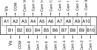
Output Cable 1
