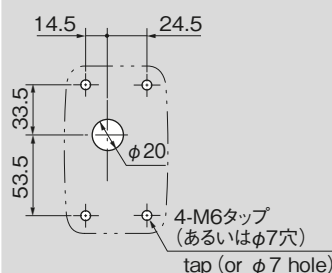
パネル穴明け寸法 Panel drilling dimensions
