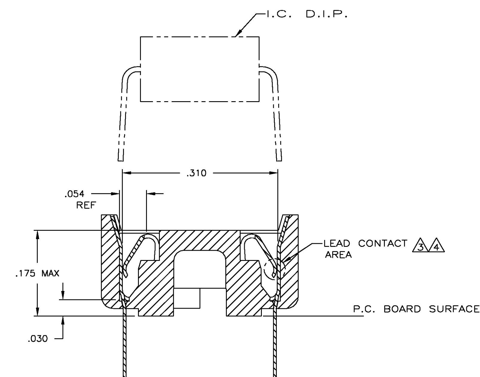
SECTION A-A SCALE 10:1
