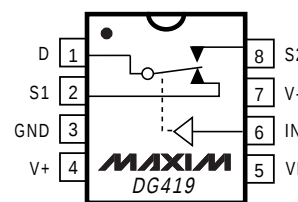
DIP/SO
