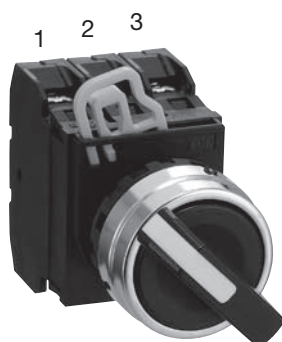
Kontaktblock Montagepositionen
