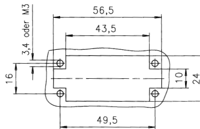
Montageausschnitt (Kontaktträger) Panel cut out (insert)
