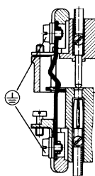
Schraubanschluss mit Drahtschutz Screw termination with wire protection
