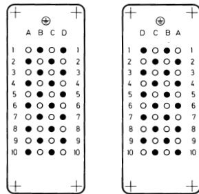
Buchseinsatz Female insert
