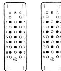
Buchseinsatz Female insert
