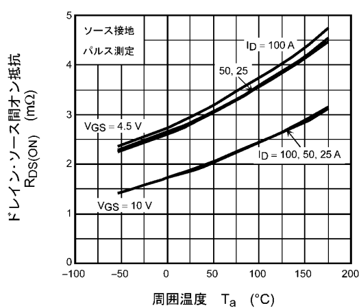
図 8.6 R_{DS(ON)} - T_a
