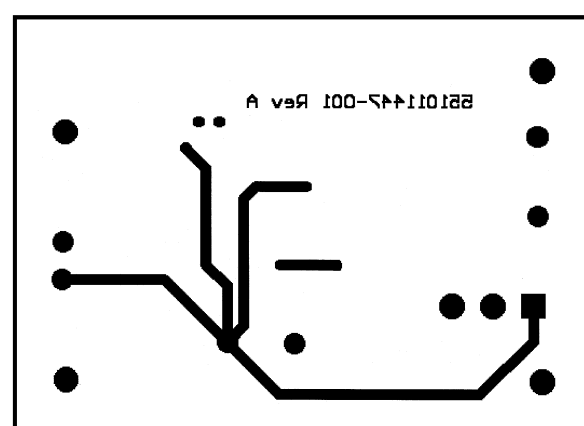
Figure 49. Bottom Layer
