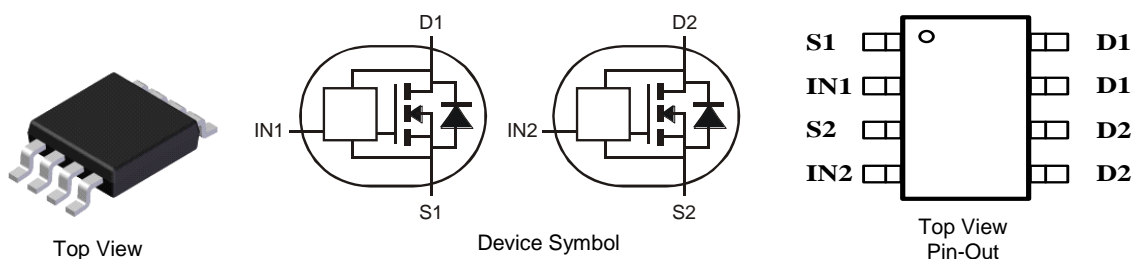
SO-8
