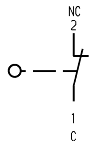
Flachstecker DIN 46244-A2.8-0.5 (EN 61058 / EN 61210)
