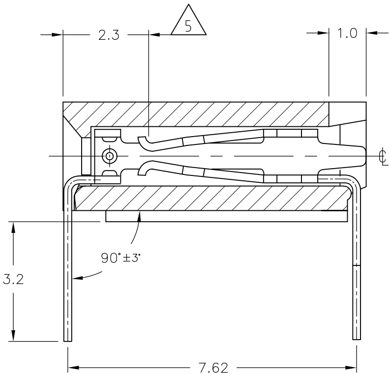
SECTION A-A
