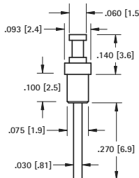
Feed-Thru
