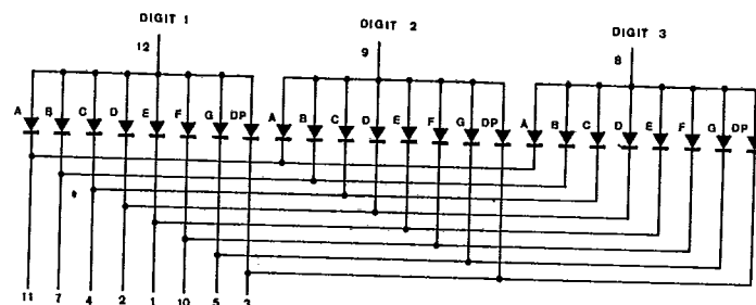
I. LTC-561
