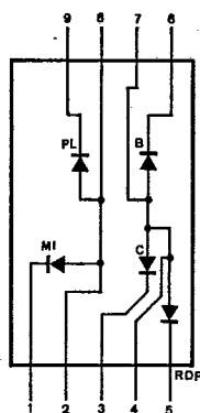
F. LTD-6x30
