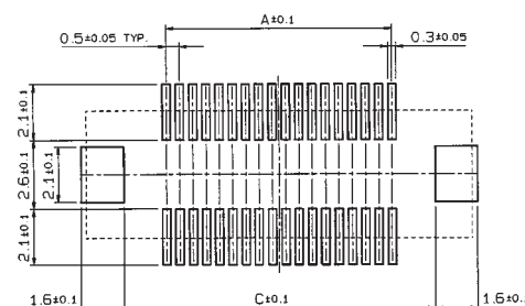
基板取り付け寸法 RECOMMENDED LAYOUT
