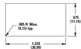
J37 Actuator
