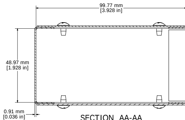
SECTION AA-AA
