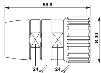
HC-..S1N..80DU , HC-..P1N..80DU
