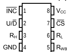
TDFN 8-Pad (ZD7, VP2) Top View
