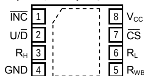
TDFN 8-Pad (ZD7, VP2) Top View
