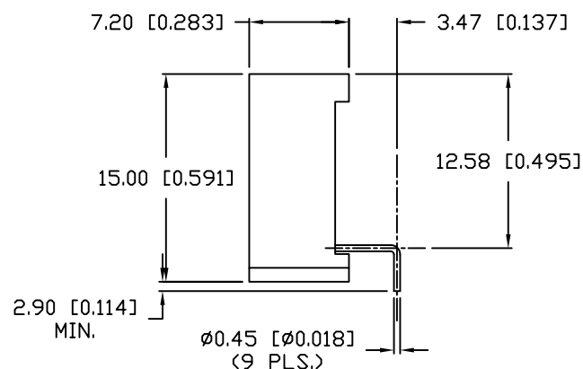
DIGIT DETAIL
