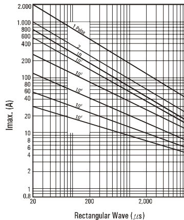
ROV20-820K – ROV20-511K
