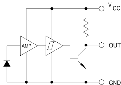
OPB685, OPB695 Buffered 10K Pull-Up
