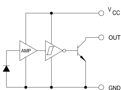
OPB688, OPB698 Inverted Open-Collector
