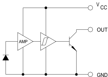
OPB686, OPB696 Buffered Open-Collector
