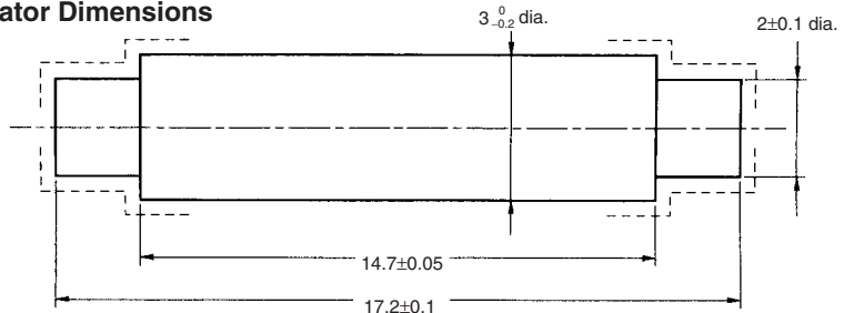
Actuator Dimensions
